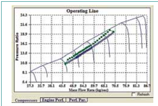
Εικόνα 7: Καμπύλη λειτουργίας συμπιεστή.
