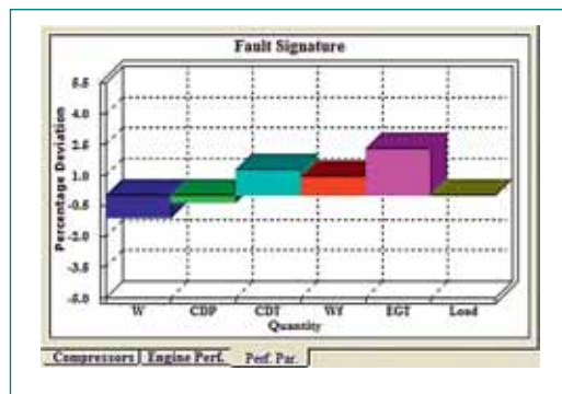
Εικόνα 8: Γραφική αναπαράσταση βασικής διαγνωστικής λειτουργίας εφαρμογής εργαστηρίου.
