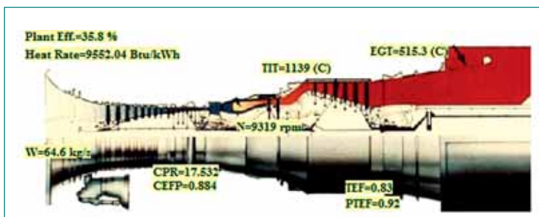
Εικόνα 3: Λειτουργικές παράμετροι πάνω στο μιμικό διάγραμμα τομής αεριοστρόβιλου.
