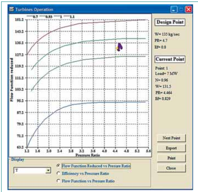
Εικόνα 6: Γραφικά αποτελέσματα προσομώησης αεροστρόβιλου (Χαρακτηριστικές καμπύλες λειτουργίας για συμπιεστή και στρόβιλο).
