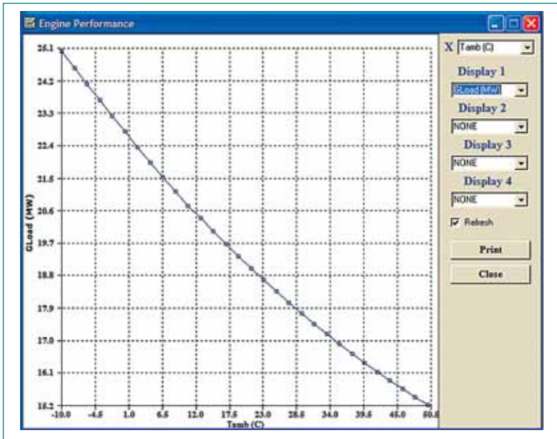
Εικόνα 5: Γραφικά αποτελέσματα προσομοίωσης αεριοστρόβιλου (Ισχύς εξόδου σε συνάρτηση με την θερμοκρασία εισαγωγής αέρα).
