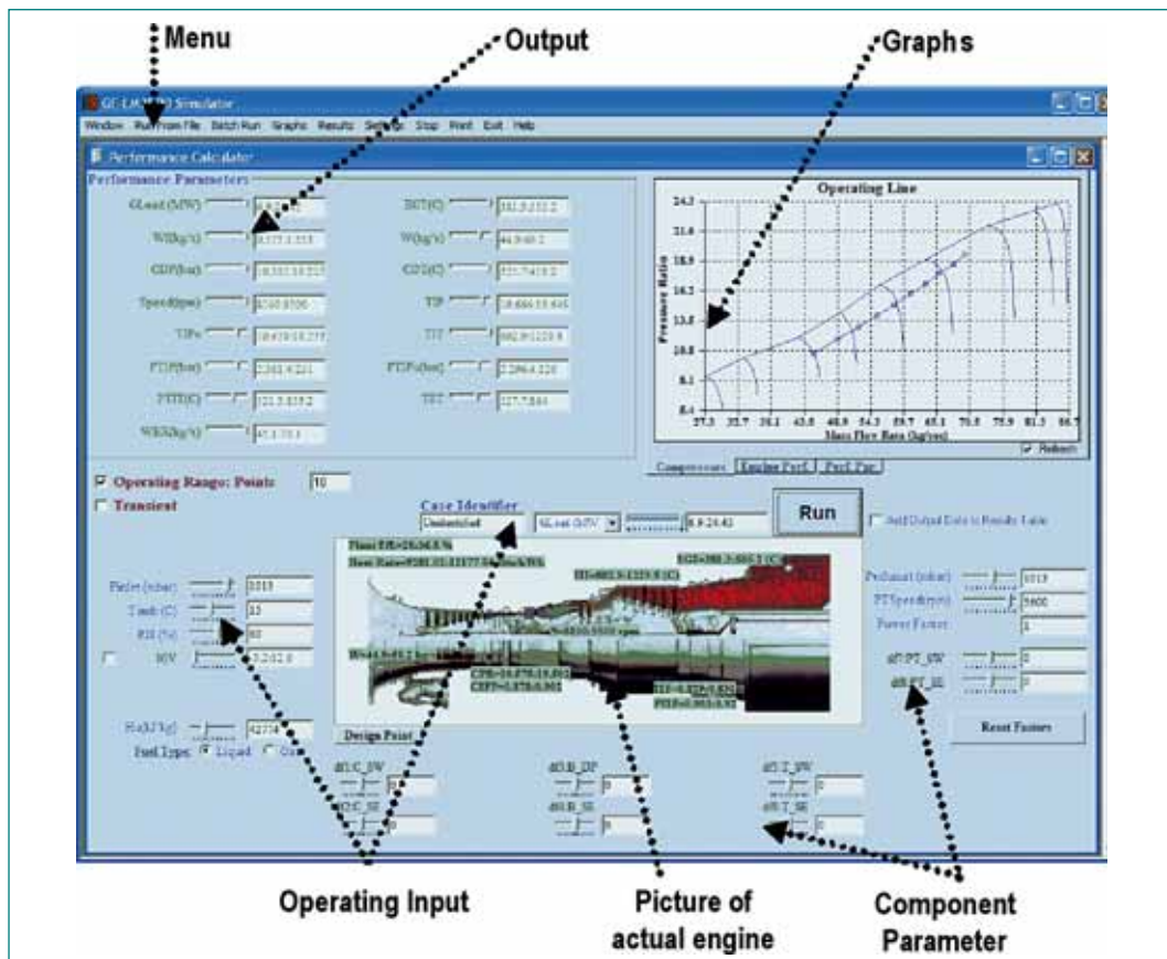
Εικόνα 2: Βασική οθόνη προσομοιωτή λειτουργίας αεριοστρόβιλου. Τμήμα εισαγωγής λειτουργικών παραμέτρων αεριοστρόβιλου.
